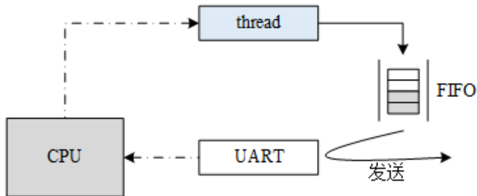
图 8.11: 中断模式驱动外设
