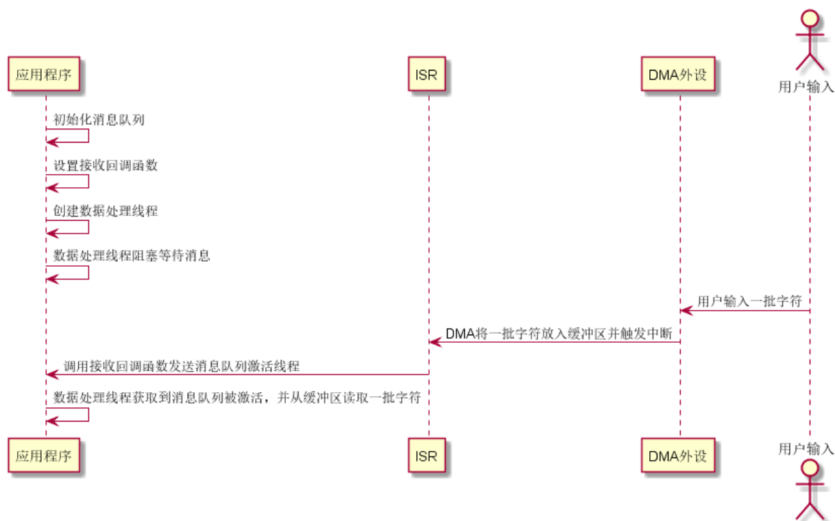
图 12.3: 串口 DMA 接收及轮询发送序列图
