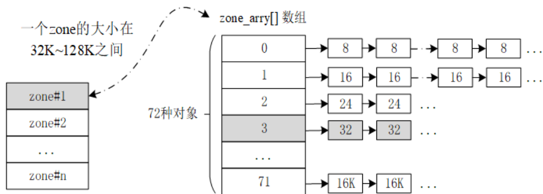
图 7.5: slab 内存分配结构图
