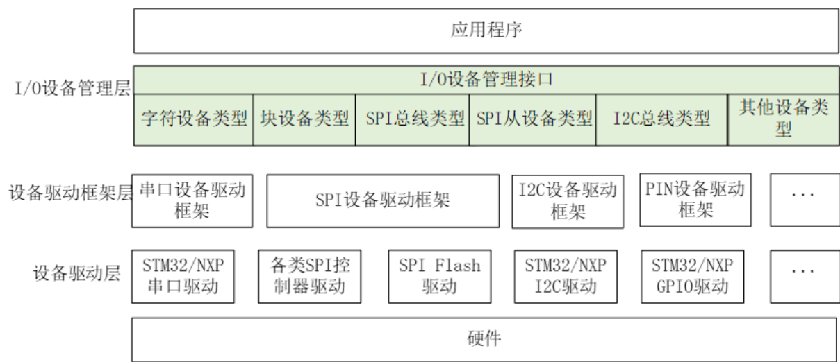
图 11.1: I/O 设备模型框架
