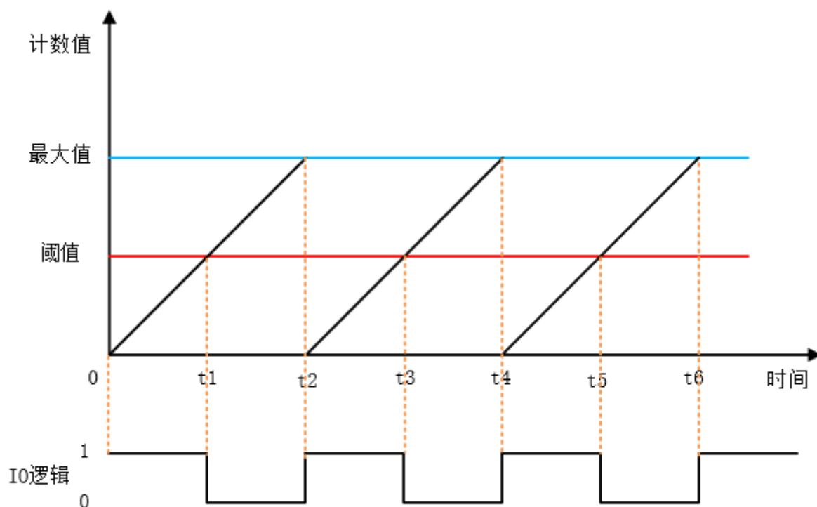
图 17.1: PWM 原理图
