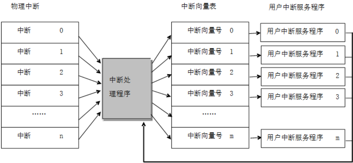
图 8.5: 中断处理过程
