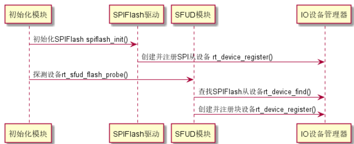
图 23.4: 注册块设备时序图
