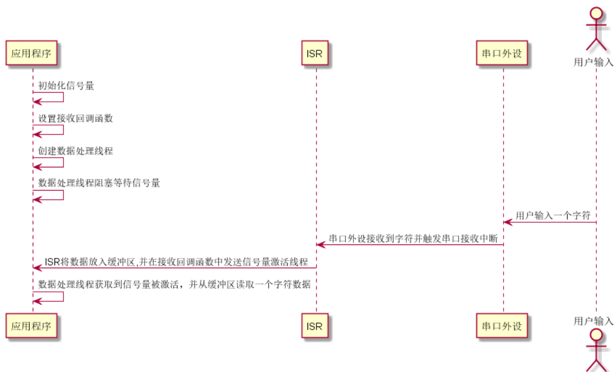
图 12.2: 串口中断接收及轮询发送序列图
