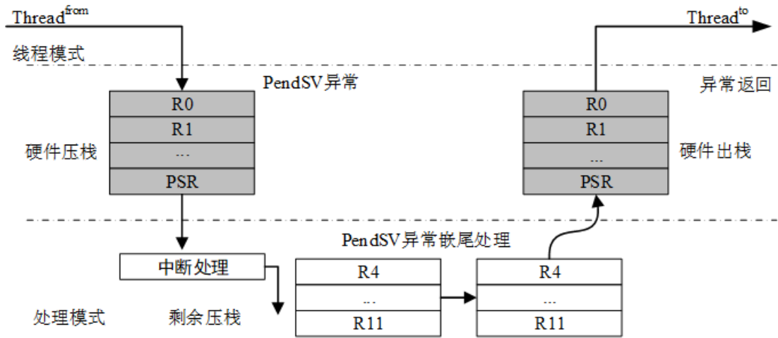
图 9.3: 中断到线程的切换
