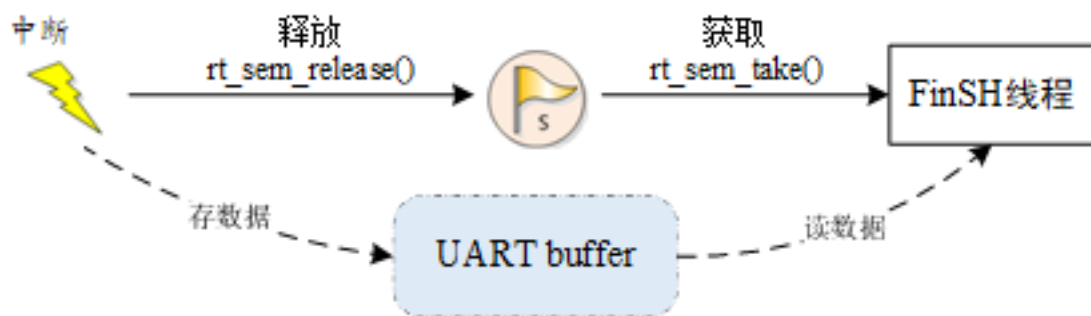
图 5.5: FinSH 的中断、线程间同步示意图
