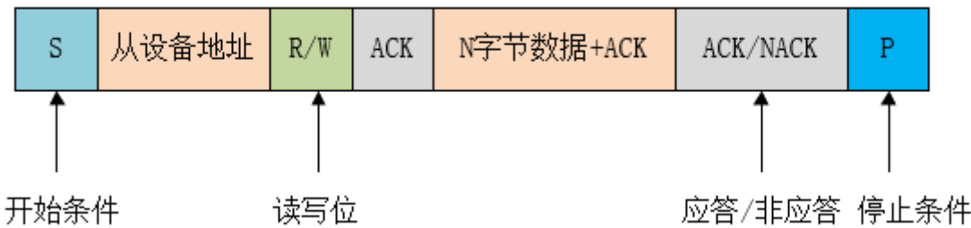
图 16.2: I2C 总线数据传输格式
