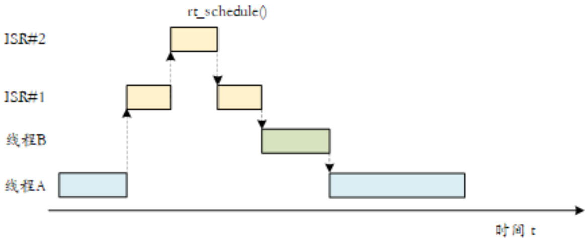
图 8.9: 中断中的线程切换
