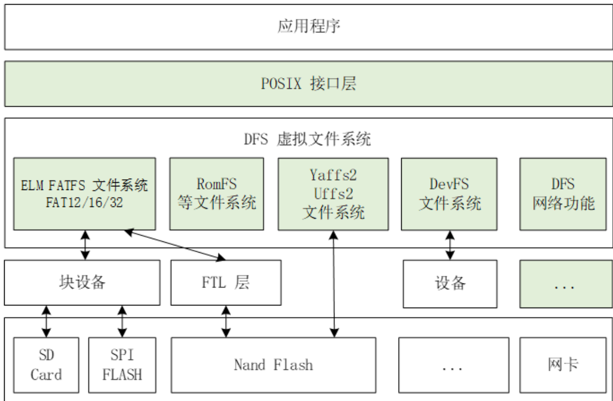
图 23.2: DFS 层次架构图
