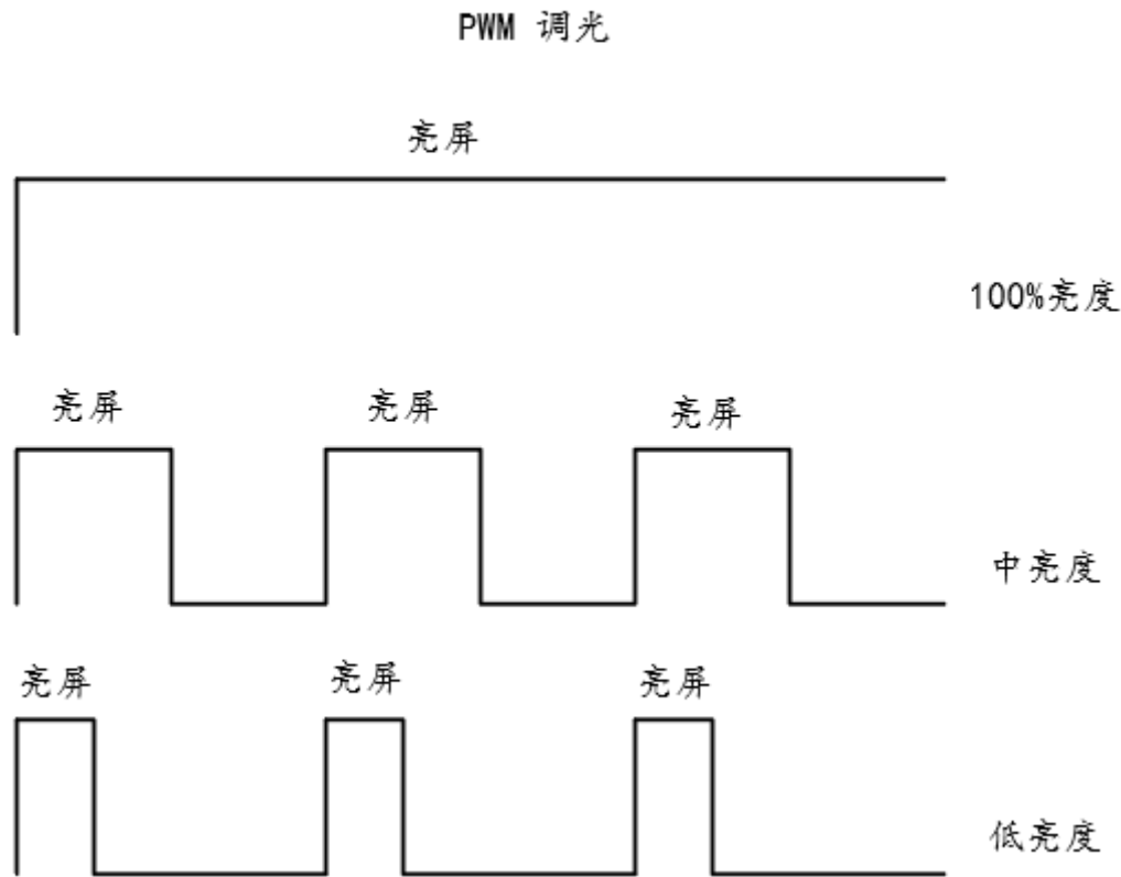
图 17.2: PWM 调节亮度
