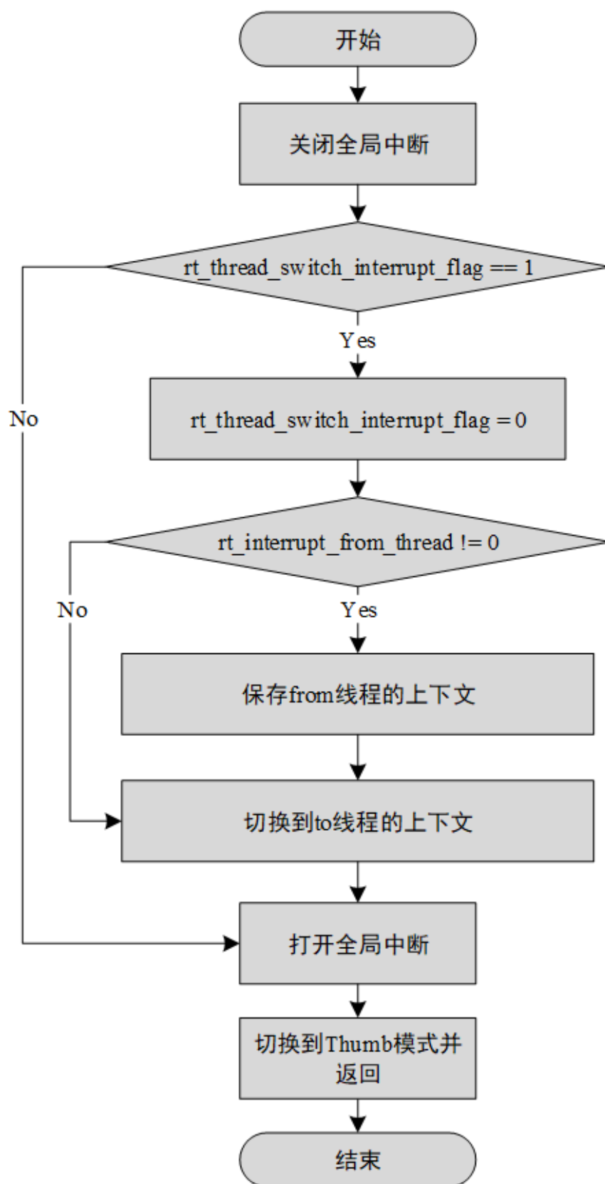
图 9.6: PendSV 中断处理
