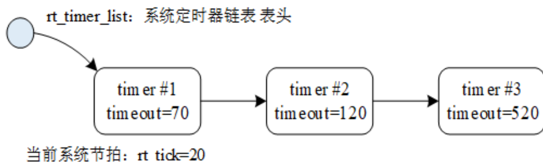
图 4.2: 定时器链表示意图
