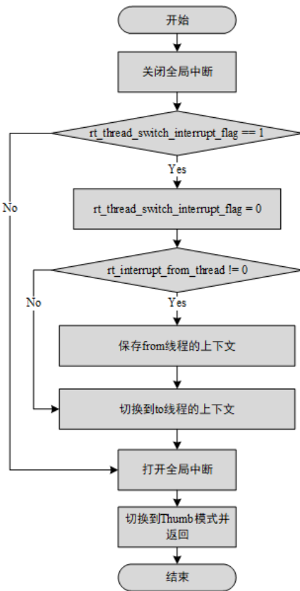
图 8.8: rt_hw_context_switch_interrupt() 函数实现流程
