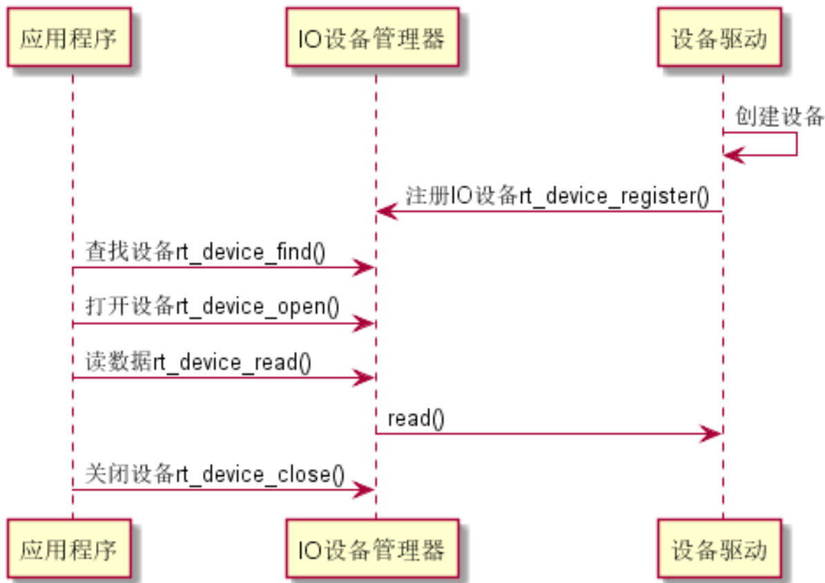
图 11.2: 简单 I/O 设备使用序列图
