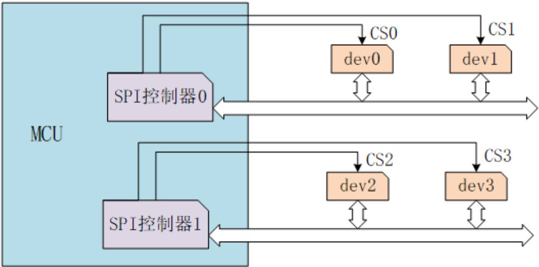
图 19.2: 一个 SPI 主设备与多个从设备连接
