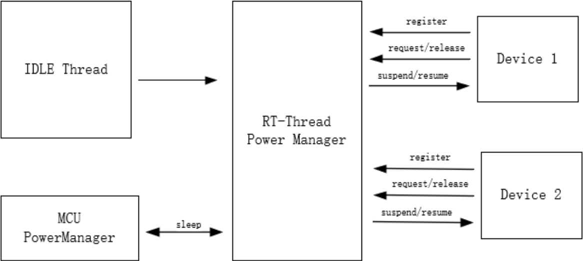
图 30.3: PM 设计架构
