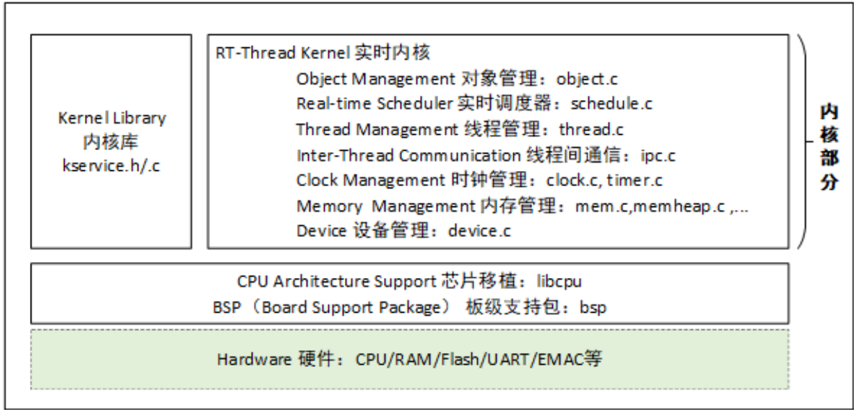
图 2.1: RT-Thread 内核及底层结构
