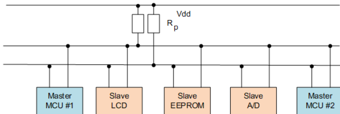
图 16.1: I2C 总线主从设备连接方式
