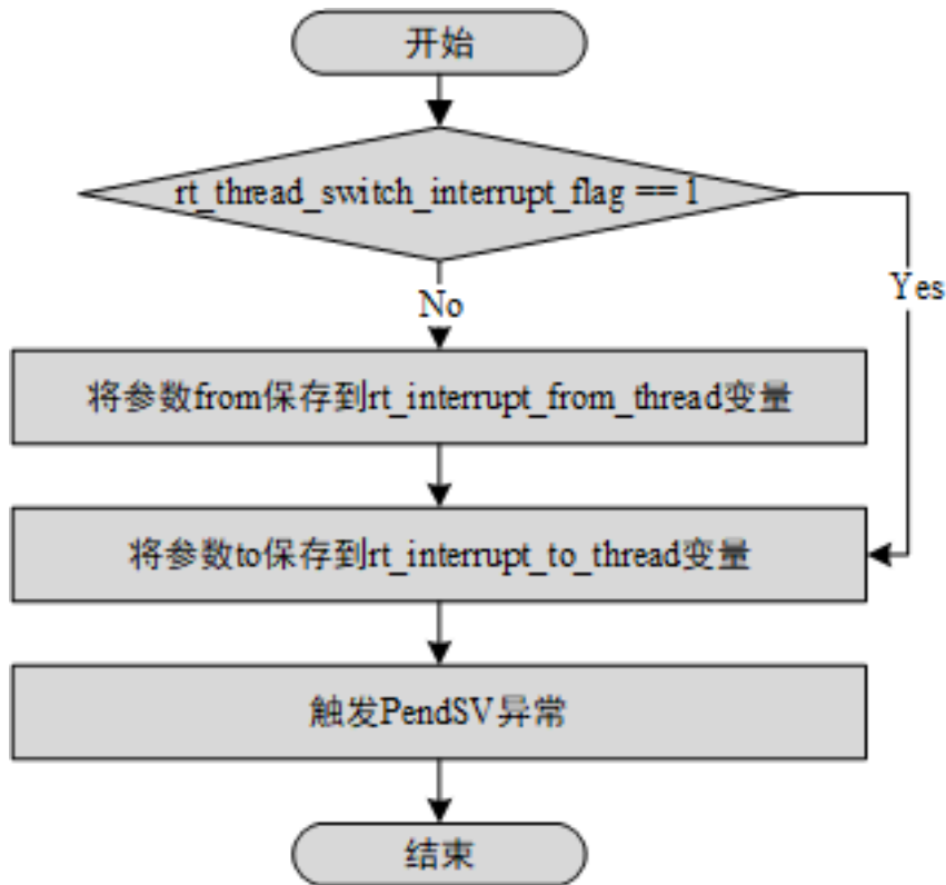
图 8.7: rt_hw_context_switch_interrupt() 函数实现流程
