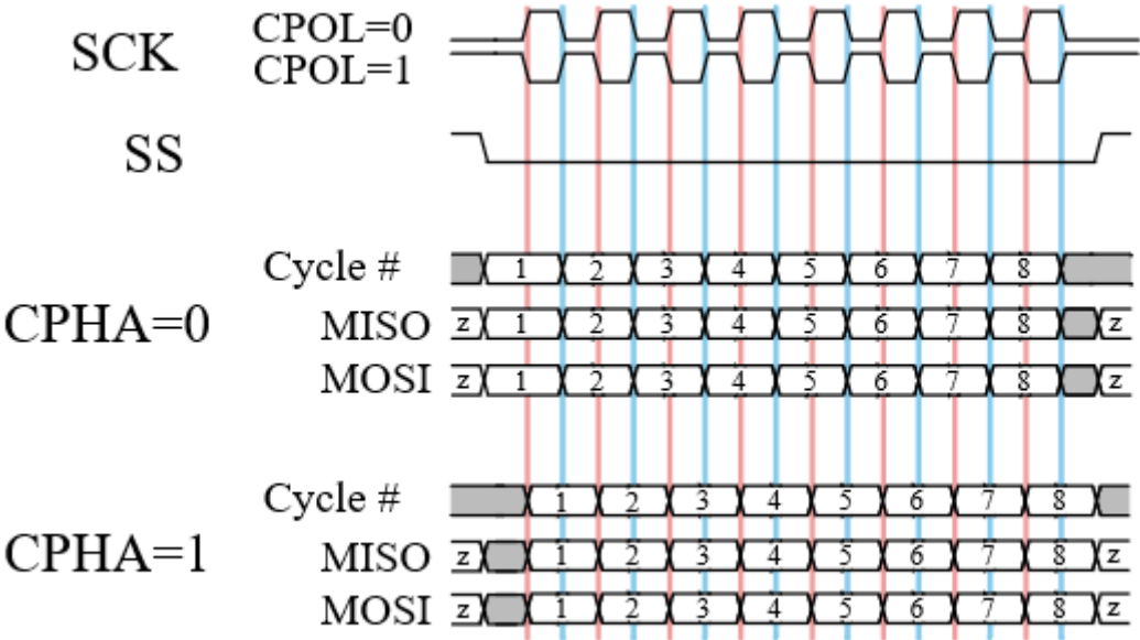
图 19.3: SPI 4 种工作模式时序图
