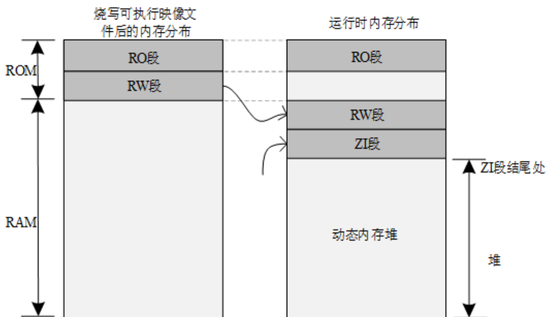
图 2.3: RT-Thread 内存分布
