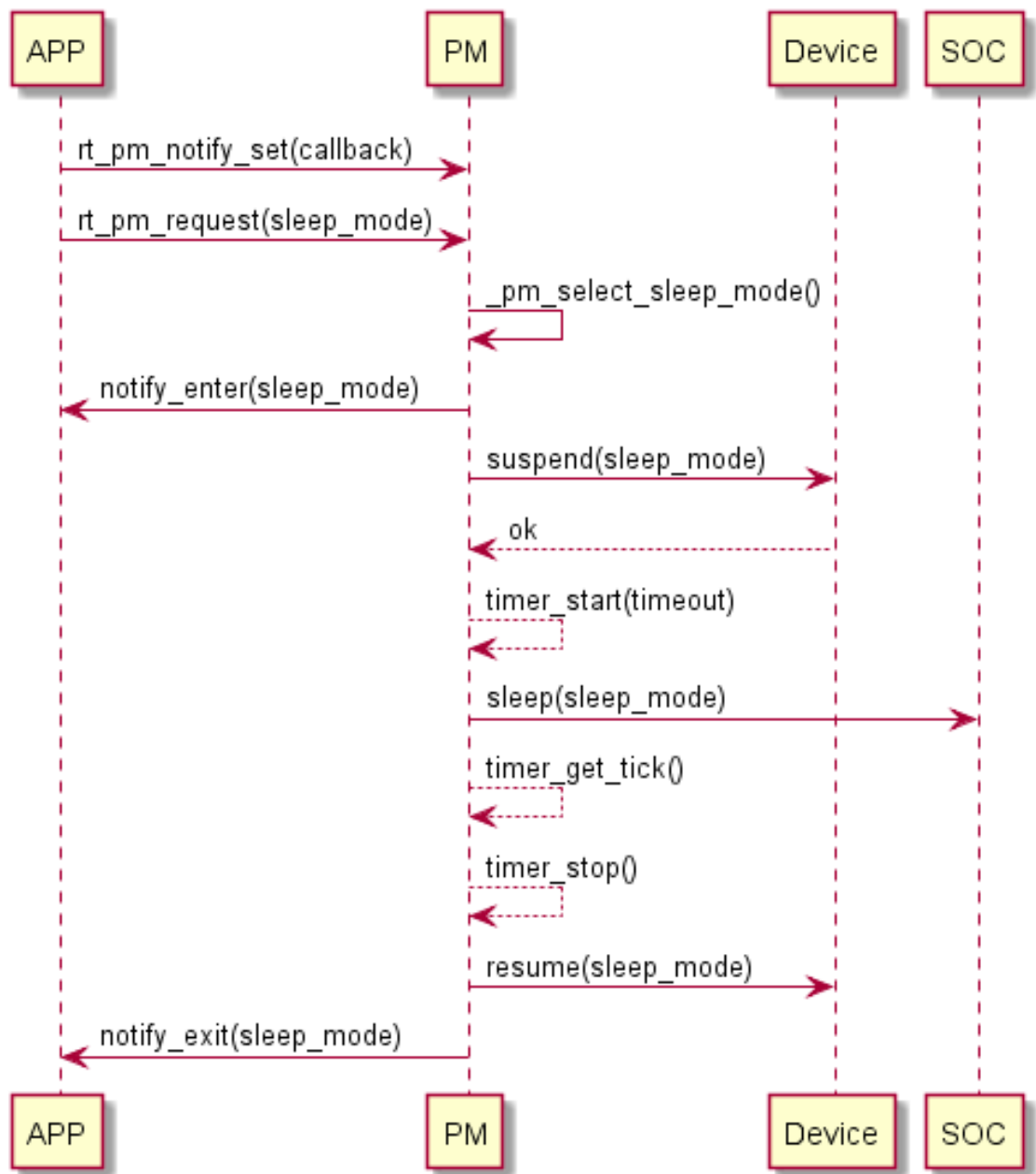
图 30.4: PM 时序图
