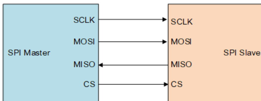
图 19.1: SPI 主设备和从设备的连接方式
