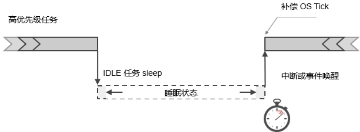
图 30.2: PM 工作原理
