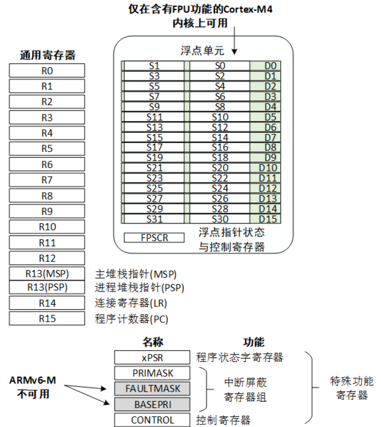
图 8.2: Cortex-M 寄存器示意图
