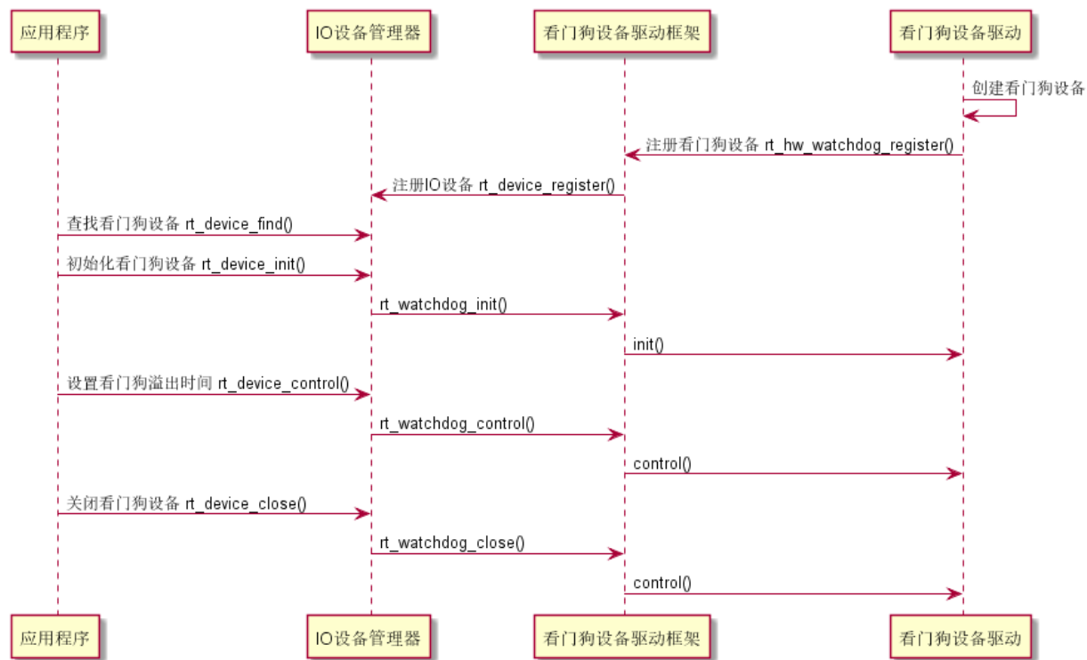
图 11.3: 看门狗设备使用序列图
