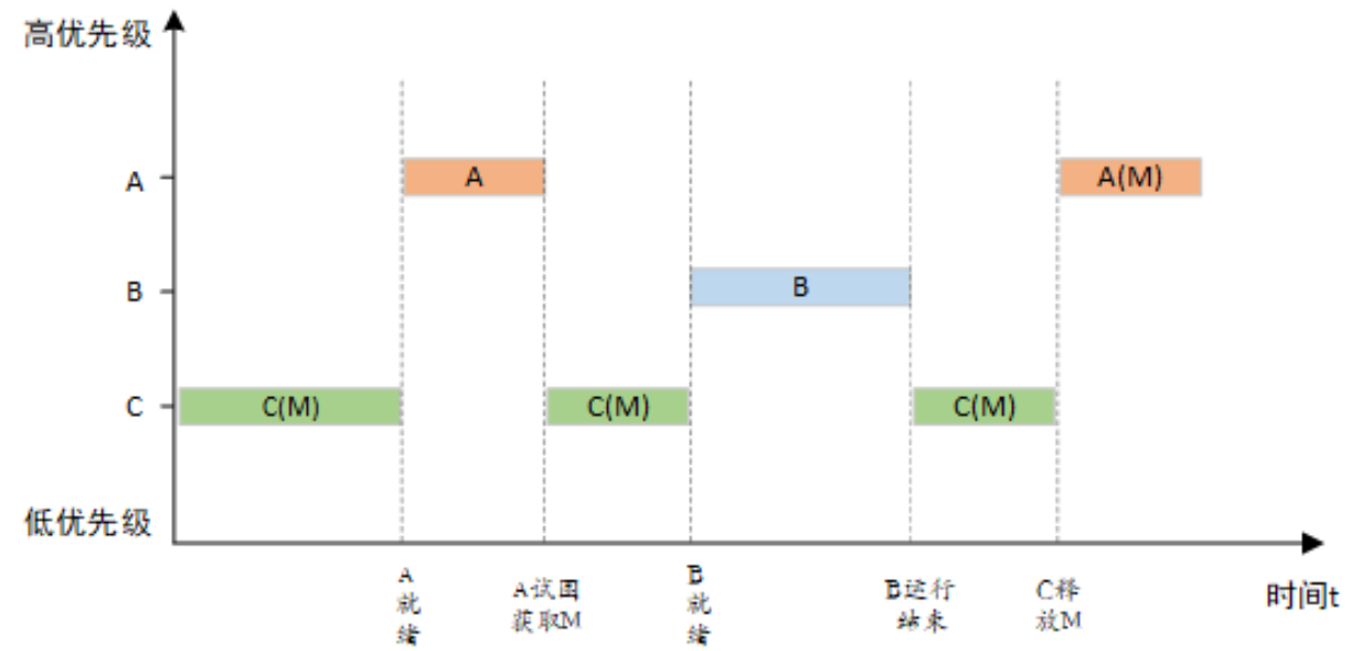
图 5.7: 优先级反转 (M 为信号量)
