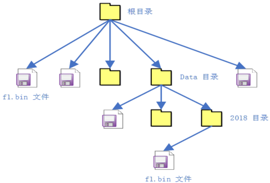
图 23.1: 目录结构图
