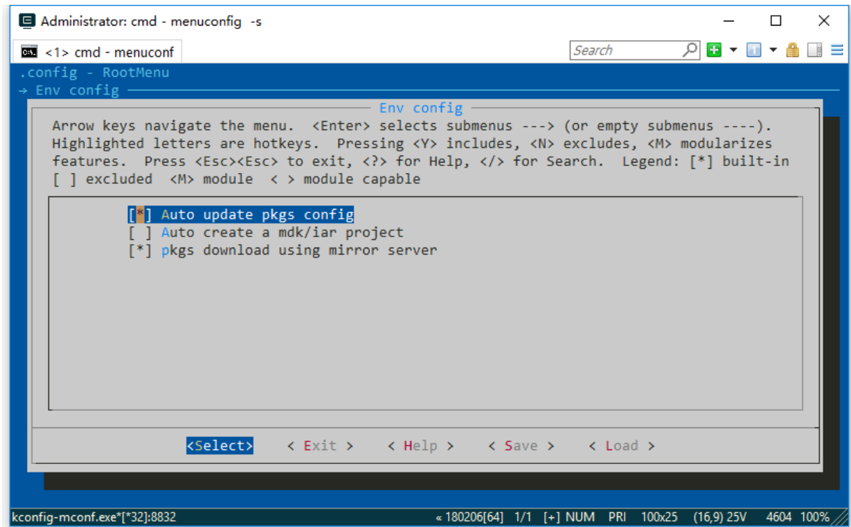
图 10.9: 配置选项
