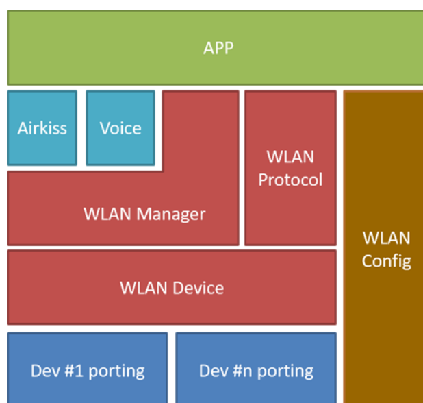
图 21.1: WIFI 框架
