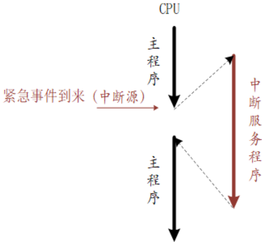
图 8.1: 中断示意图
