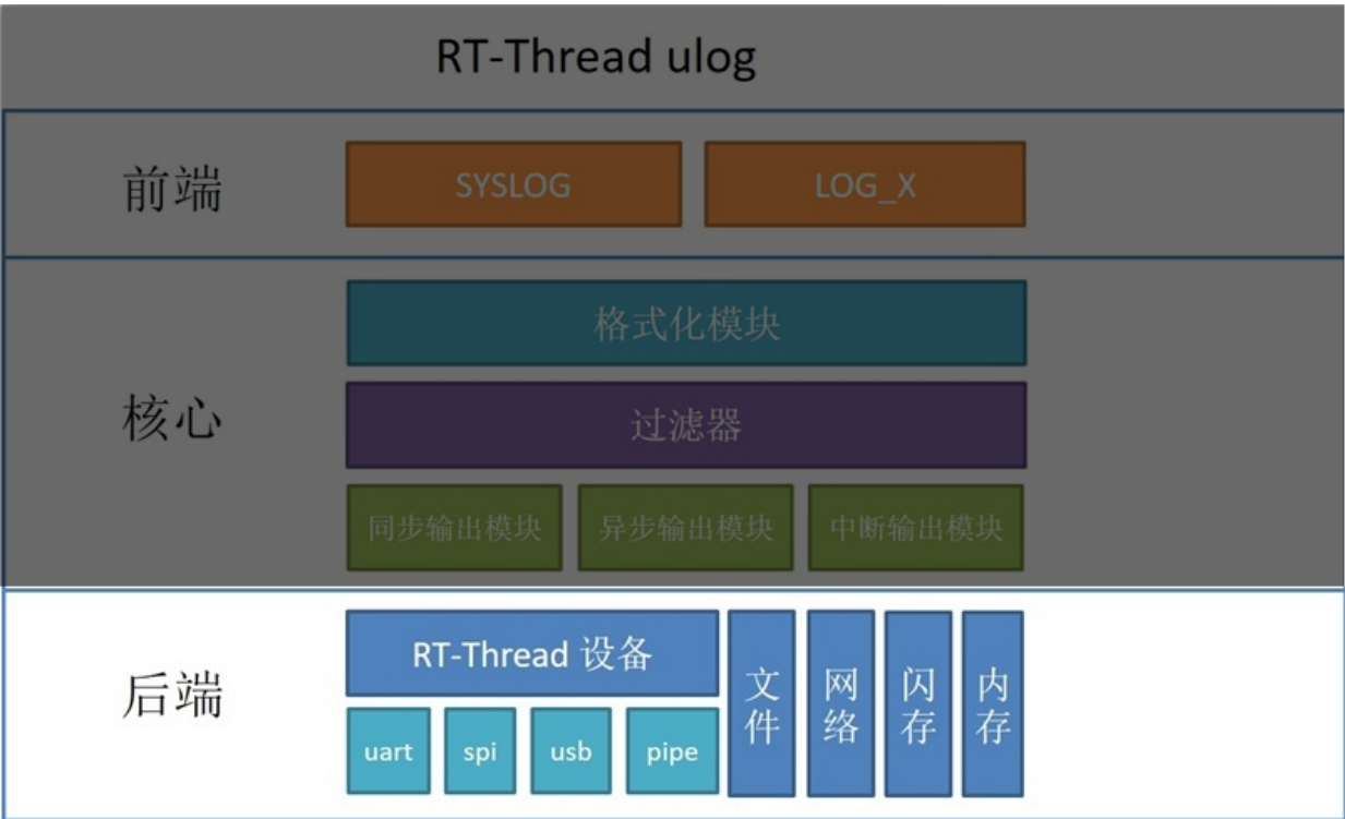
图 26.6: ulog 框架
