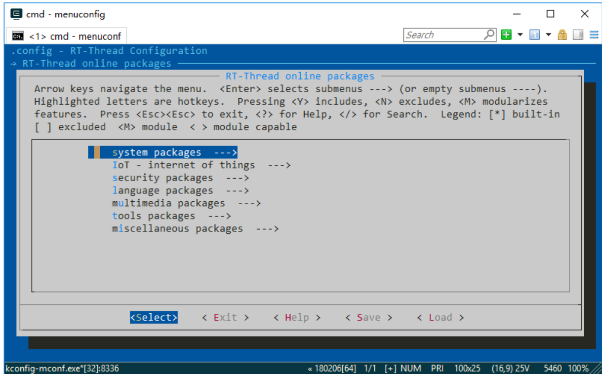
图 10.7: 软件包分类
