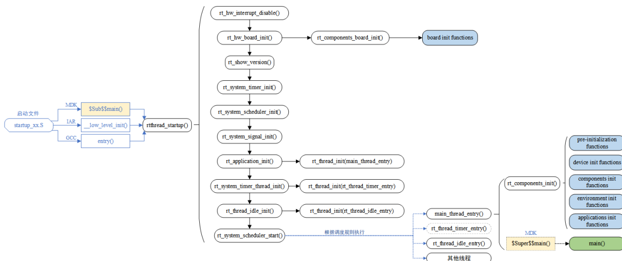
图 2.2: 启动流程
