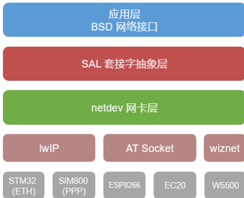
图 25.1: 网络框架图
