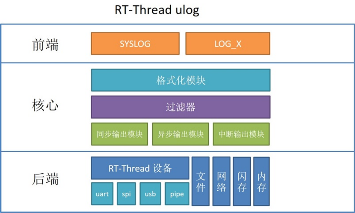
图 26.1: ulog 框架
