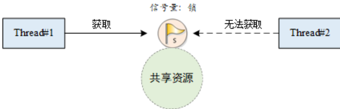
图 5.4: 锁
