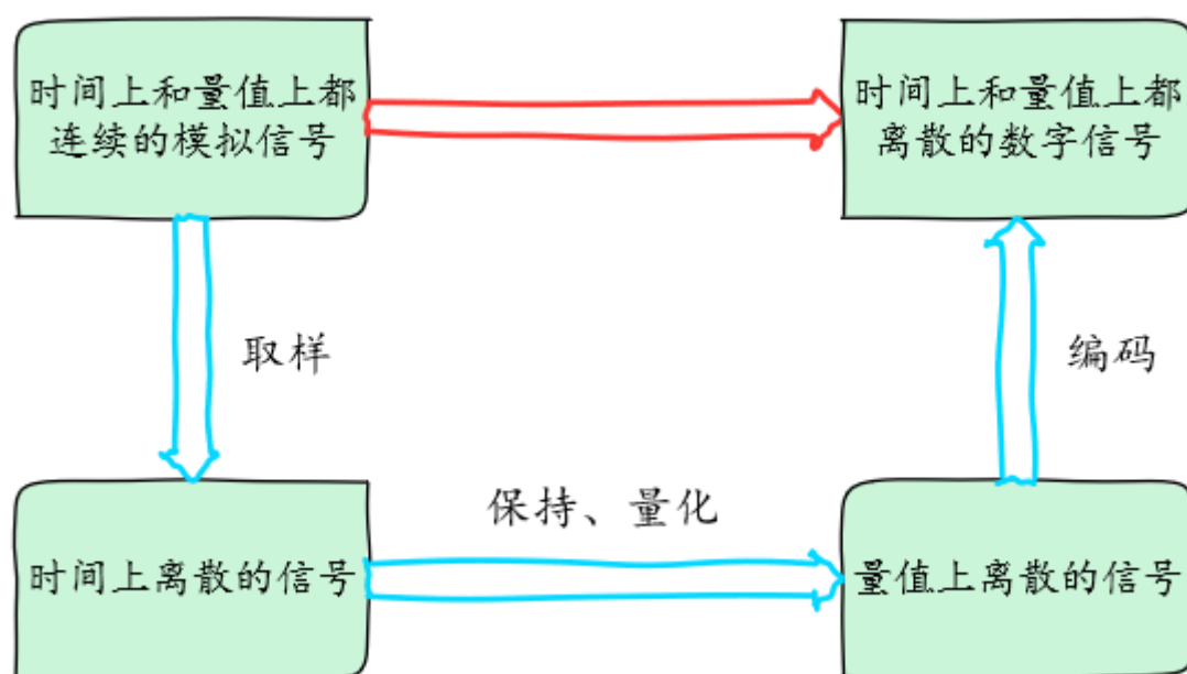
图 14.1: ADC 转换过程
