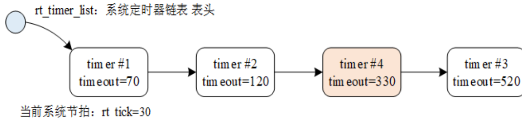
图 4.3: 定时器链表插入示意图
