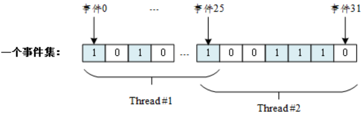
图 5.12: 多事件接收示意图
