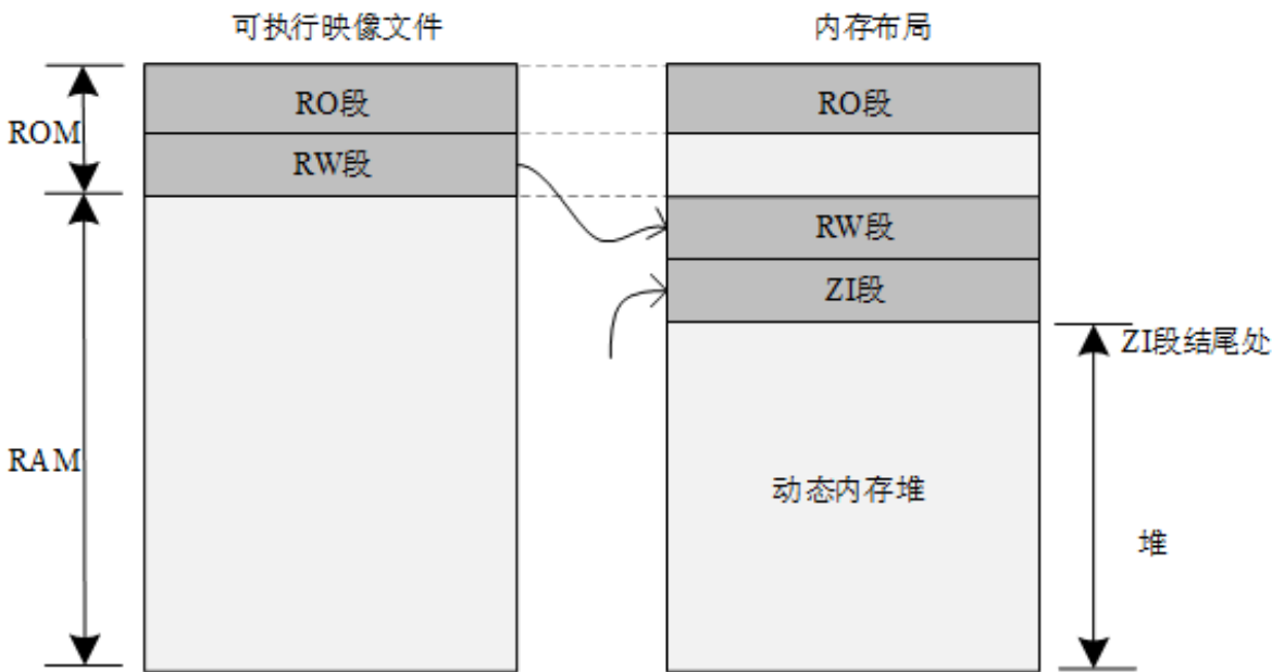
图 7.1: RT-Thread 内存分布
