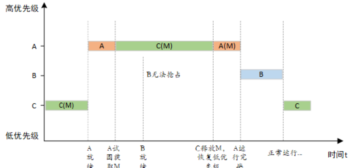
图 5.8: 优先级继承 (M 为互斥量)
