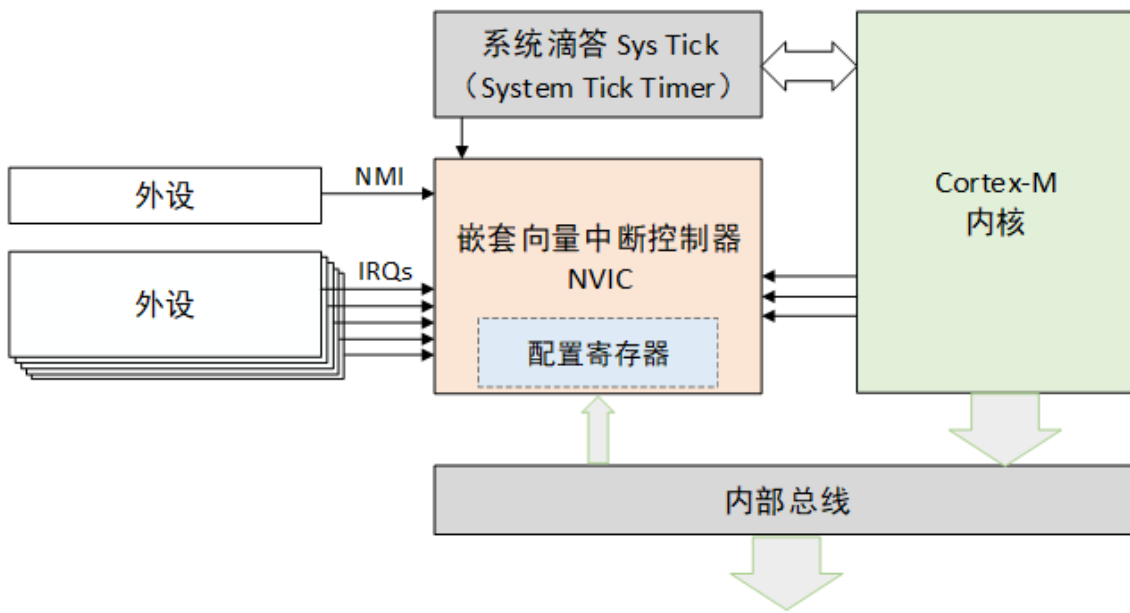
图 8.4: Cortex-M 内核和 NVIC 关系示意图
