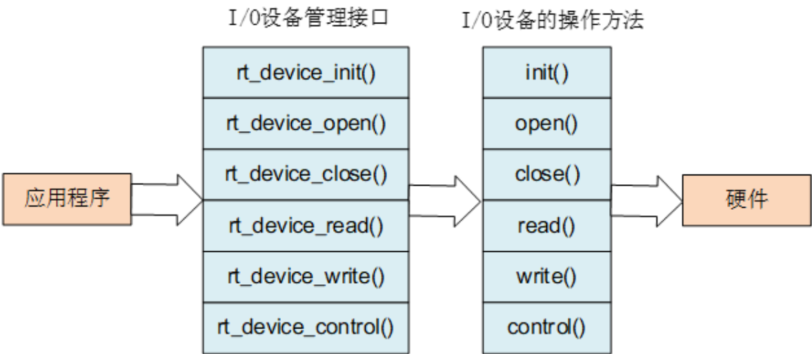
图 11.6: I/O 设备管理接口与 I/O 设备的操作方法的映射关系
