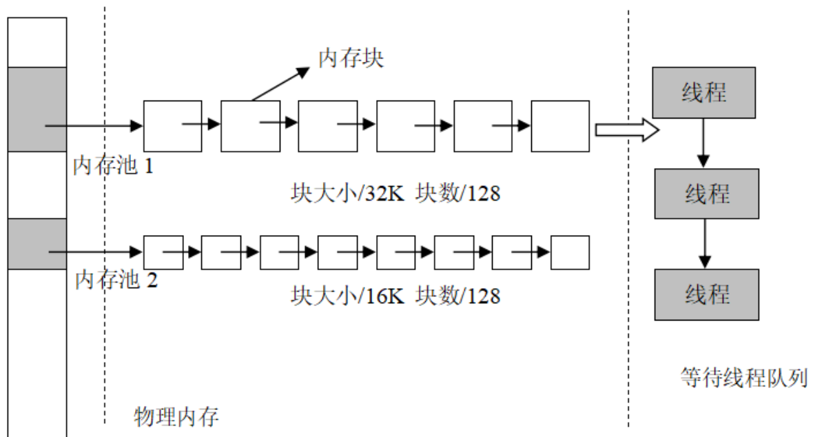
图 7.9: 内存池工作机制图
