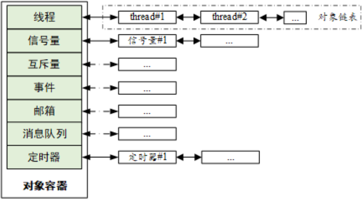
图 2.4: RT-Thread 的内核对象容器及链表
