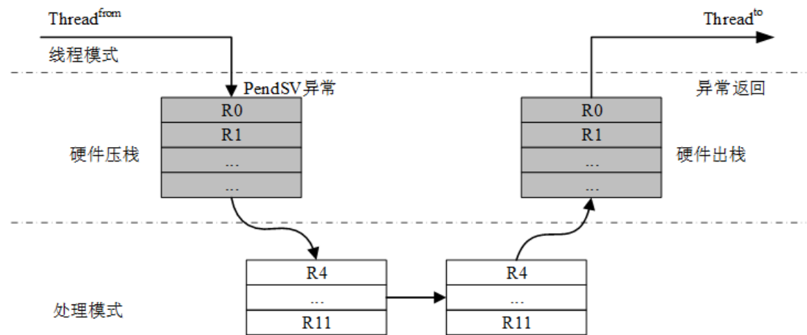
图 9.2: 线程之间的上下文切换
