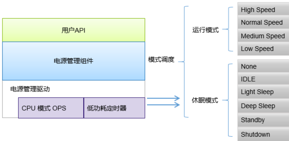
图 30.1: PM 组件概略图
