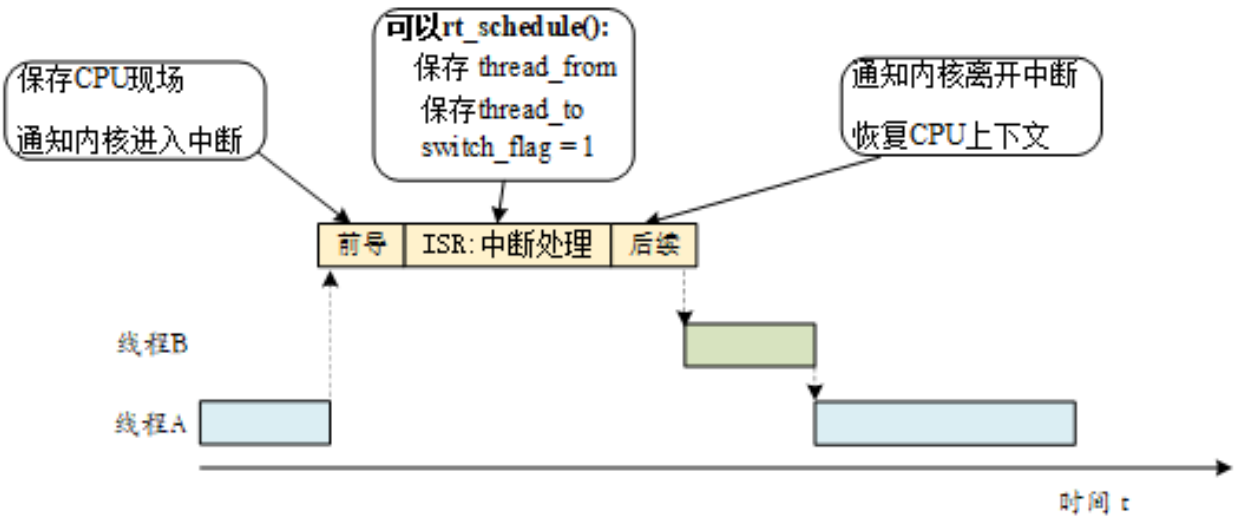
图 8.6: 中断处理程序的 3 部分
