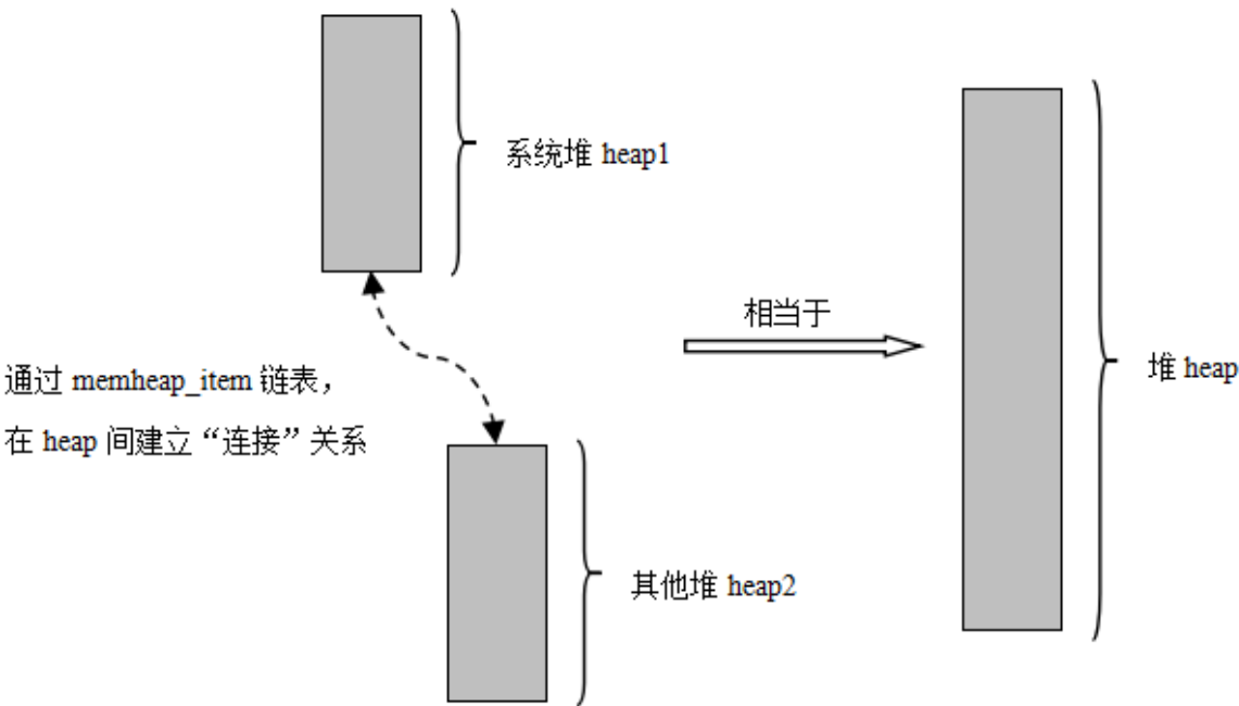
图 7.6: memheap 处理多内存堆
