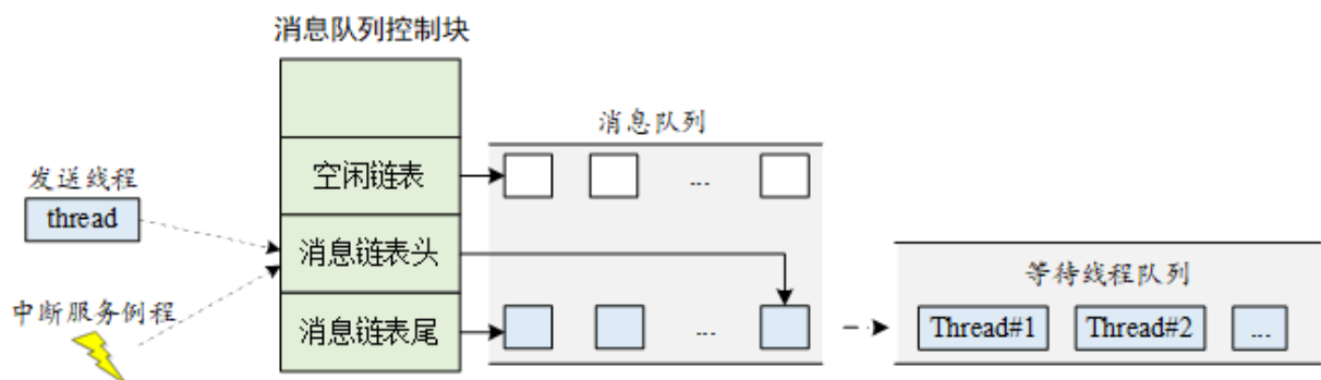
图 6.3: 消息队列工作示意图
