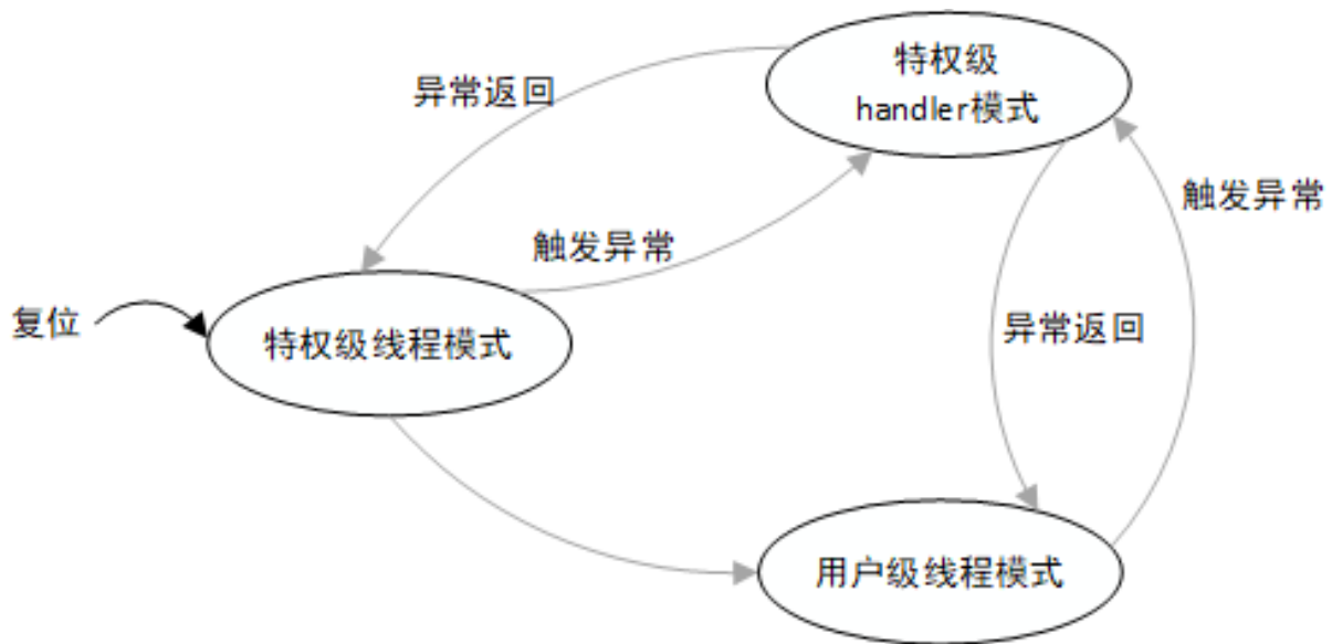
图 8.3: Cortex-M 工作模式状态图
