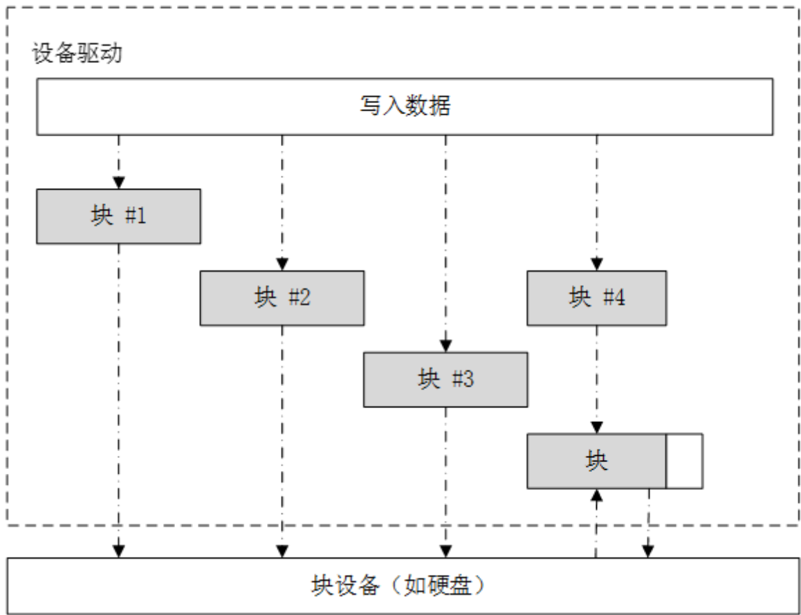
图 11.5: 块设备
