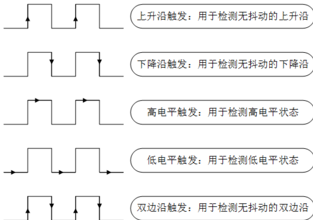
图 13.1: 5 种中断触发模式
