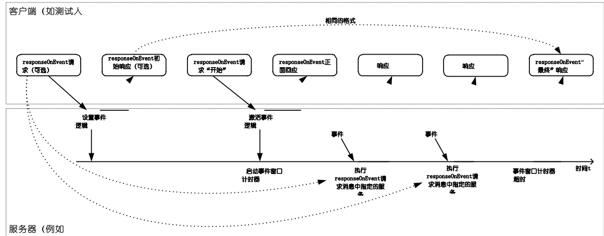
图10 - ResponseOnEvent服务 - 客户端和服务行为
