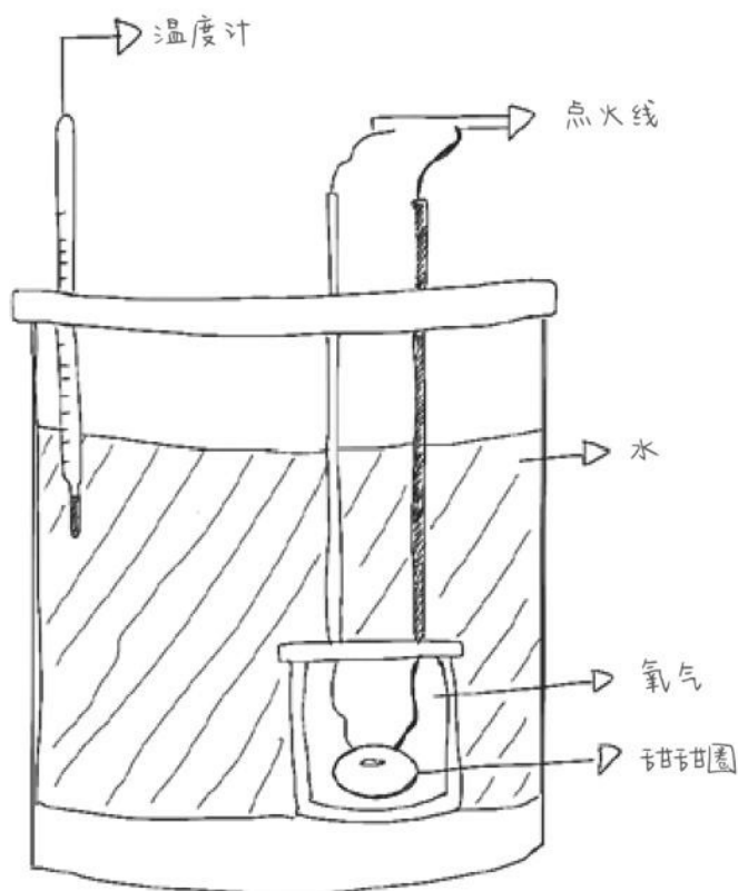
图3-25 甜甜圈的热量计算装置
