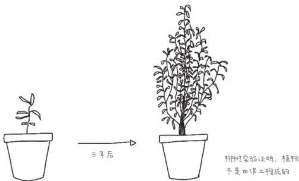
图1-1 柳树实验
