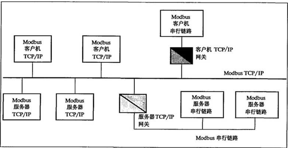
图 2 Modbus TCP/IP 通信结构
