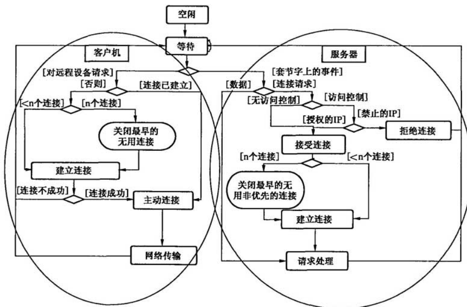
图 8 TCP 连接管理操作图
