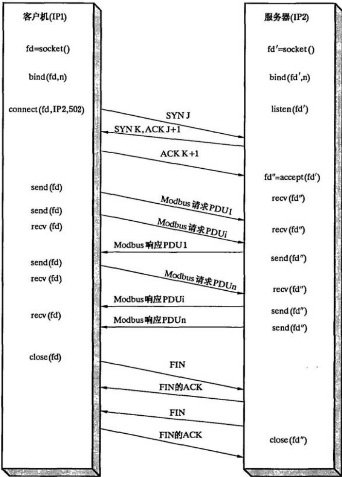
图 11 Modbus 信息交换
