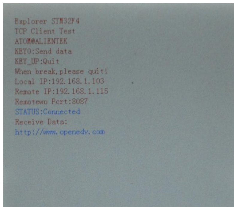
图 4.3.4 LCD 显示接收到的数据
