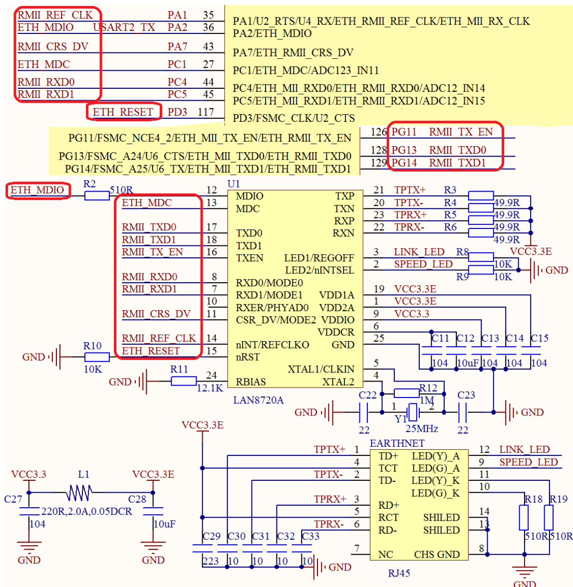
图 1.2.1 LAN8720 以太网原理图
