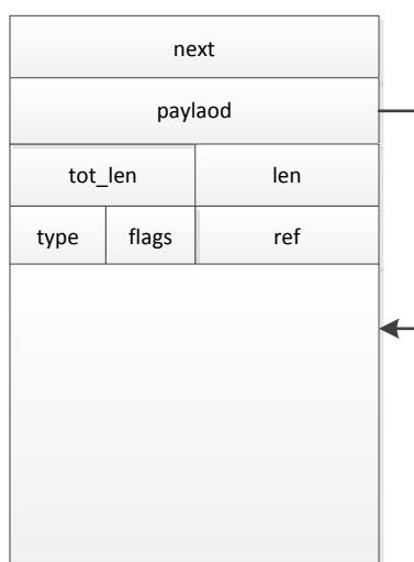
图 1.3.4.1 PBUF_RAM 类型 pbuf
