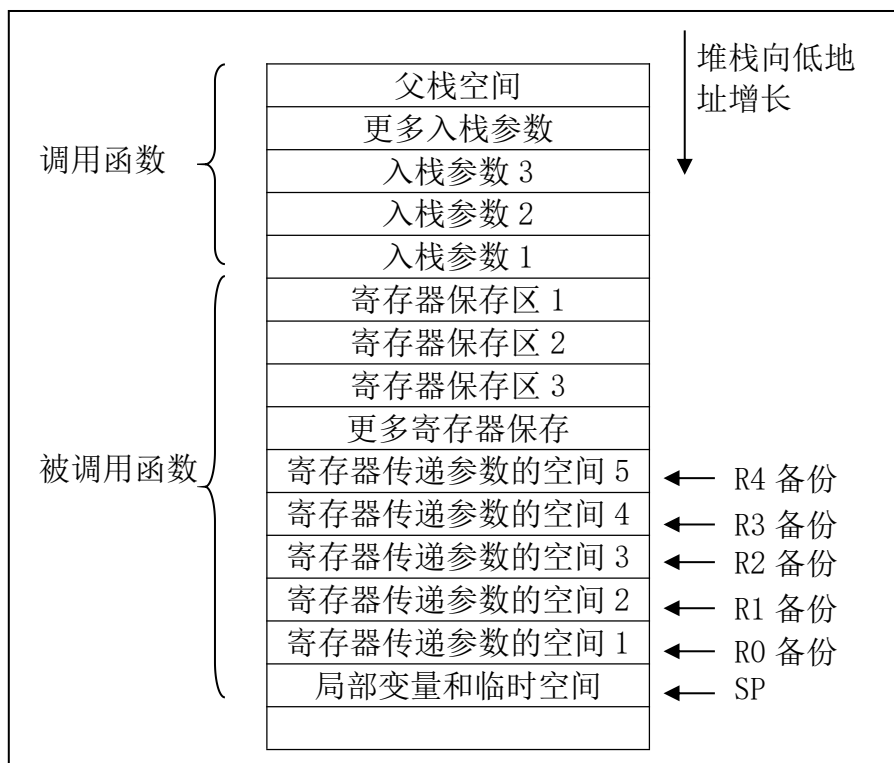
图 6-1 堆栈帧
